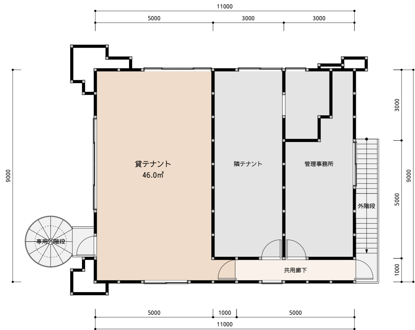
二階平面図
