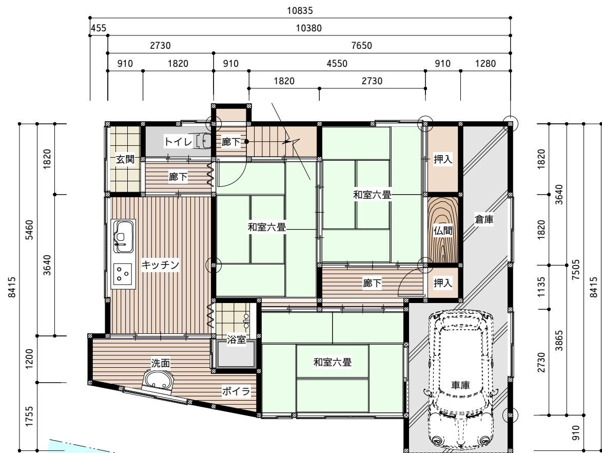
一階平面図 (S=1/100)
